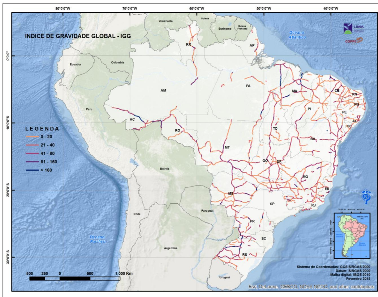
Figura 8. Índice de Gravidade Global (IGG), para os segmentos de rodovia analisados
