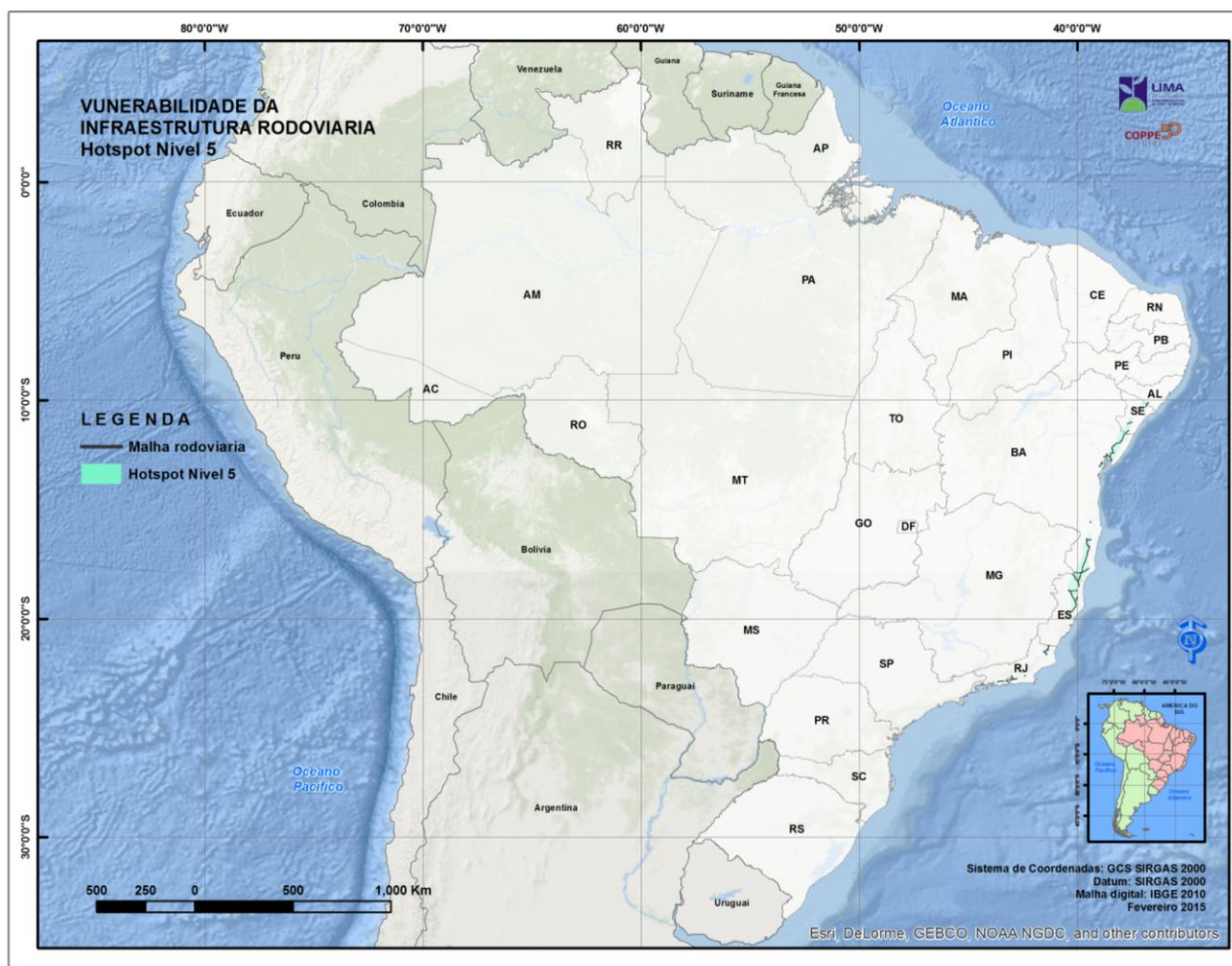
Figura 6. Malha rodoviária no hotspot Nível 5 (N5), definido pelo ensemble dos hotspots para Temp7dias e RX1day, dos modelos Eta/HadGEM2-ES e Eta/MIROC5, RCP 4.5 e RCP 8.5
