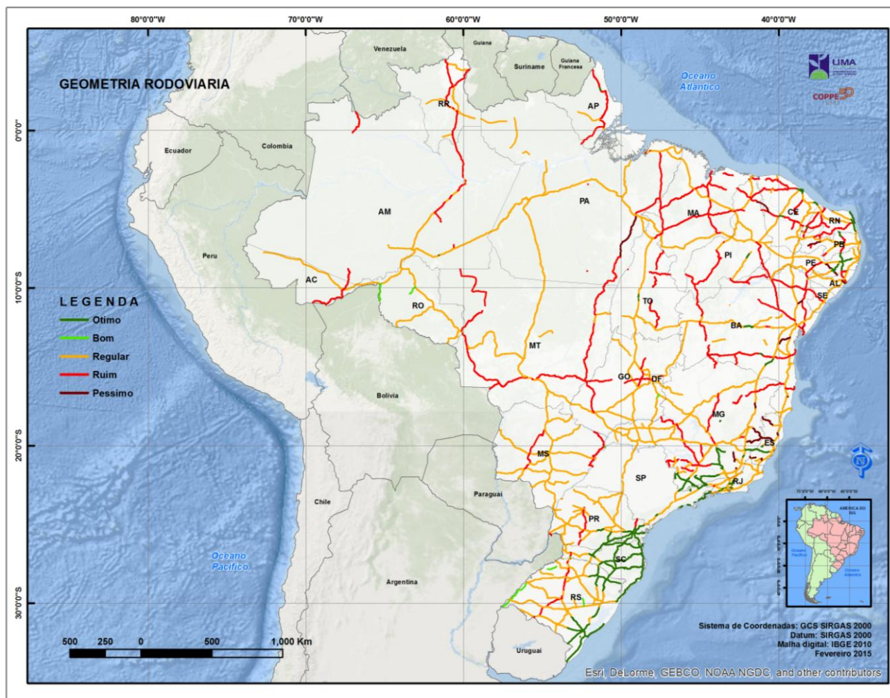
Figura 9. Classificação da Geometria para os segmentos de rodovia analisados
