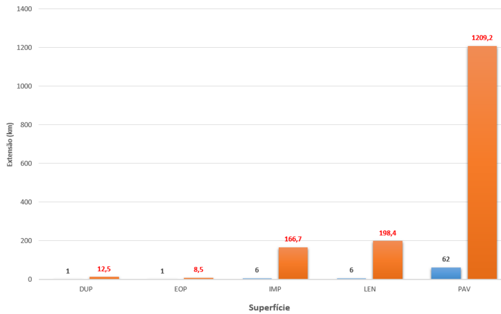
Figura 38. Extensão (km) da malha rodoviária por tipo de superfície de alta e muito alta vulnerabilidade, para o período presente
