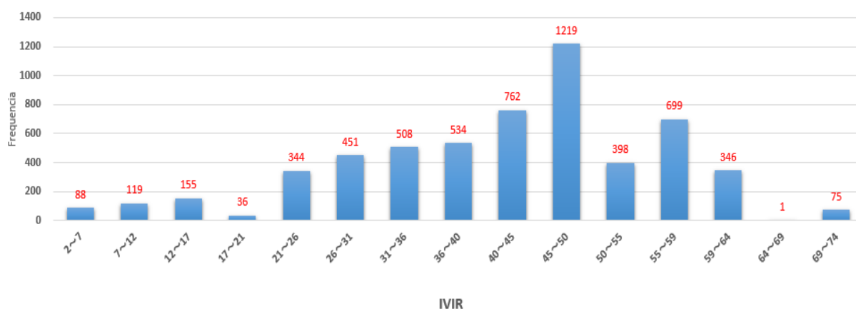
Figura 30. Histograma de distribuição do Índice de Vulnerabilidade da Infraestrutura Rodoviária (IVIR) presente
