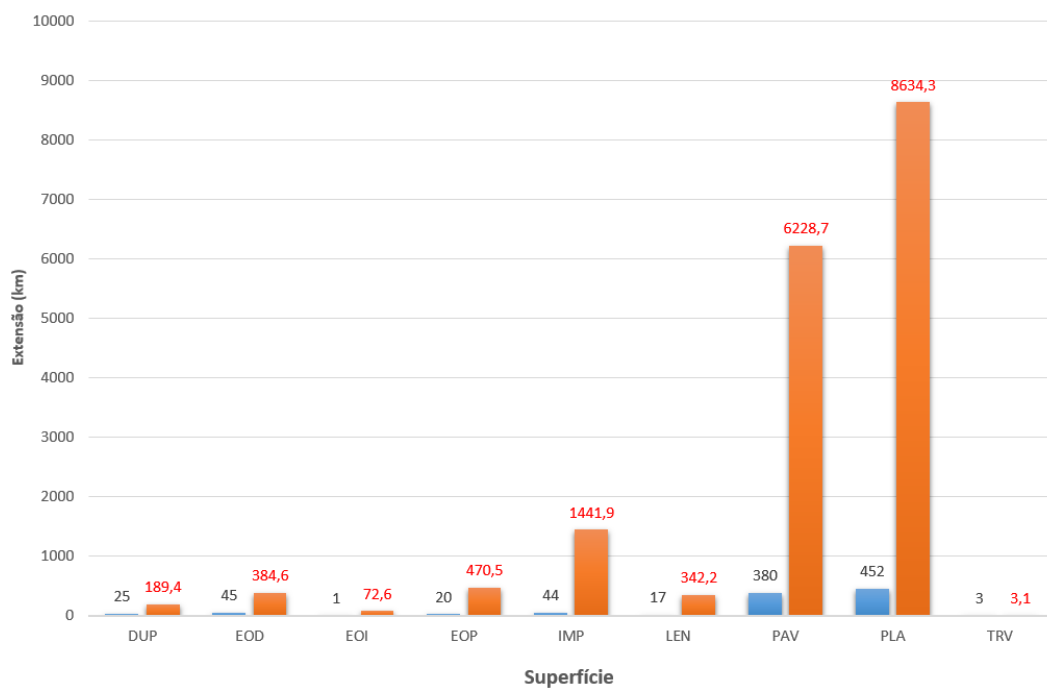
Figura 39. Extensão (km) da malha rodoviária por tipo de superfície de alta e muito alta vulnerabilidade, para o período futuro
