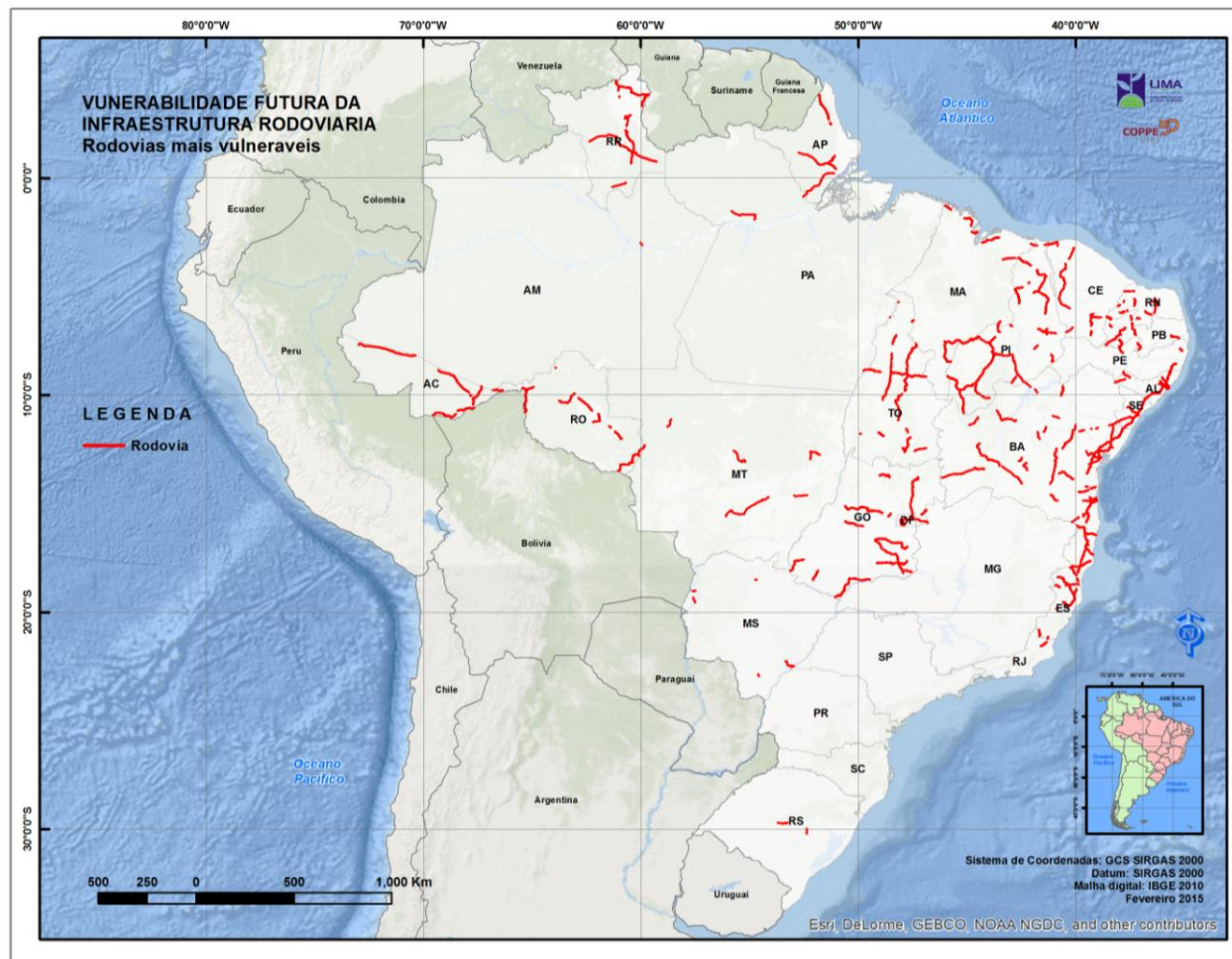
Figura 36. Segmentos de rodovias mais vulneráveis no futuro, com base no Índice de Vulnerabilidade da Infraestrutura Rodoviária presente – IVIRp
