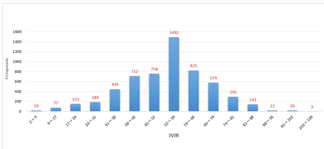
Figura 31. Histograma de distribuição do Índice de Vulnerabilidade da Infraestrutura Rodoviária (IVIR) futuro (período de integração 2011-2040)
