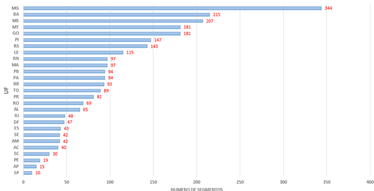
Figura 12. Número de segmentos analisados para IRI e IGG, por Unidade da Federação e Distrito Federal
