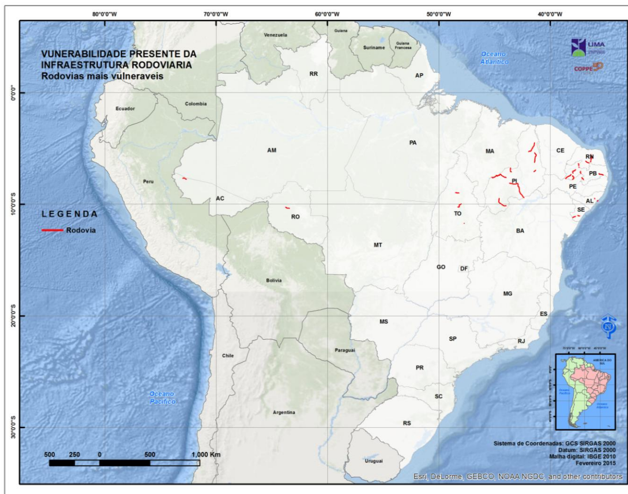
Figura 35. Segmentos de rodovias mais vulneráveis no presente, com base no Índice de Vulnerabilidade da Infraestrutura Rodoviária presente – IVIRp
