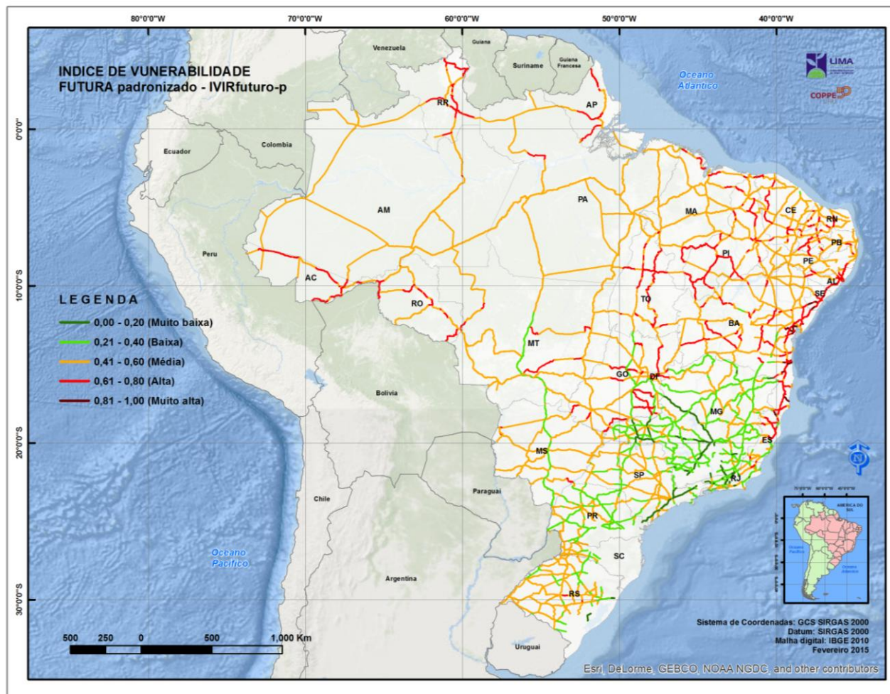
Figura 33. Índice de Vulnerabilidade da Infraestrutura Rodoviária futuro padronizado (IVIRfuturo-p)
